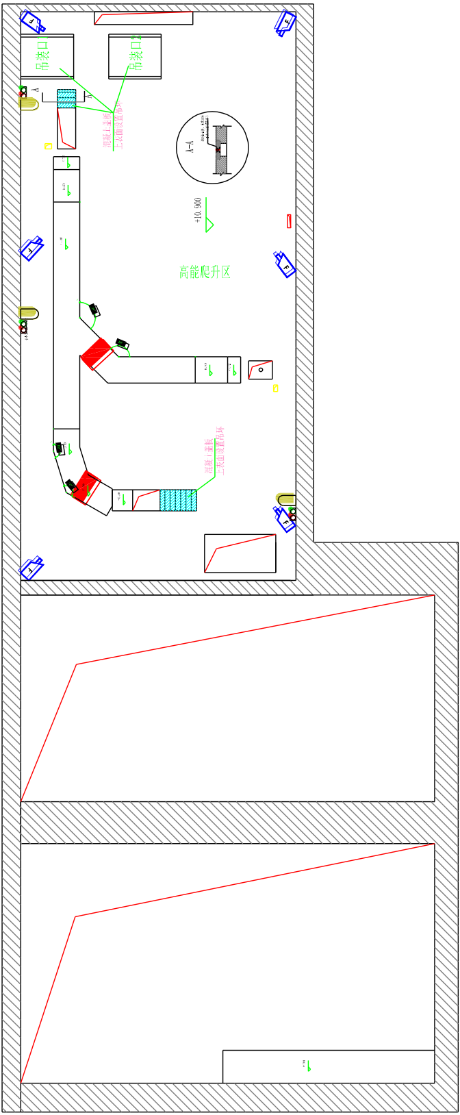
图 4.1.2-14 质子重离子机房内安全联锁设施安装点位（三层）
