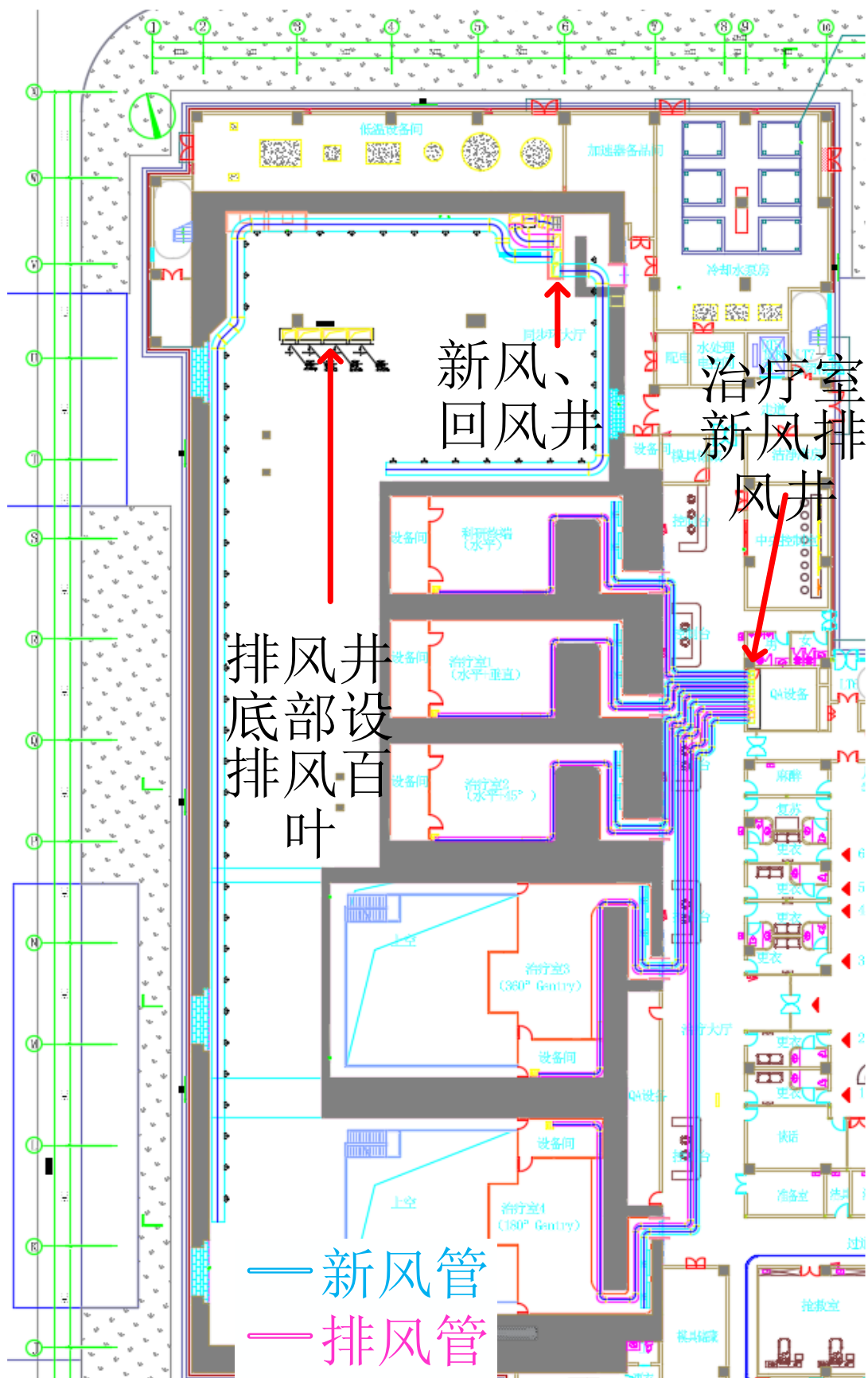
图 4.1.2-17 质子重离子机房通排风管道示意图（一层）
