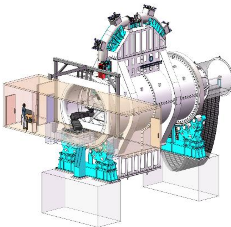
图3.2.1-14 治疗室3中360° Gantry治疗终端效果示意图
