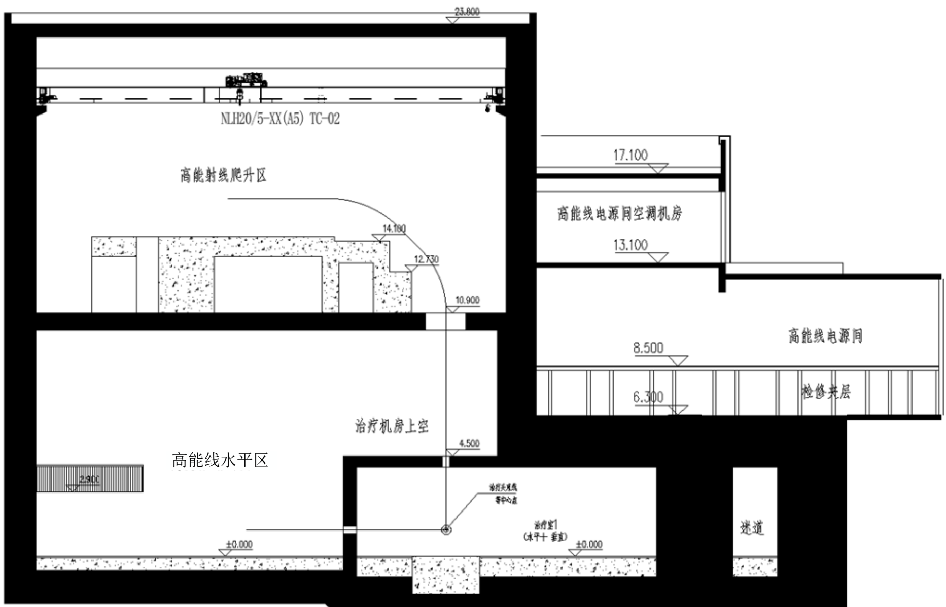
图 1.2.5-10 重离子质子中心剖面布置图
