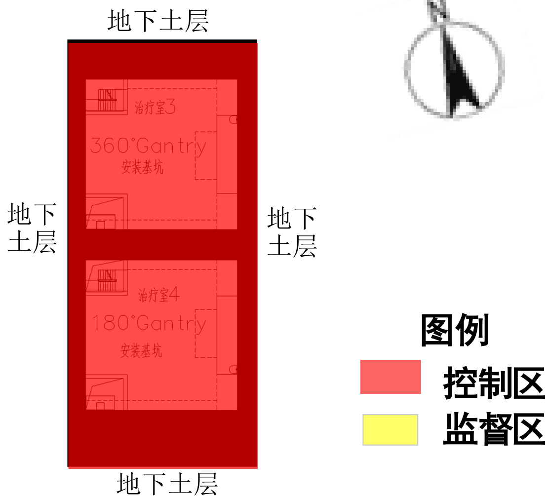
图 4.1.1-1 质子重离子机房辐射工作场所分区图（负一层）
