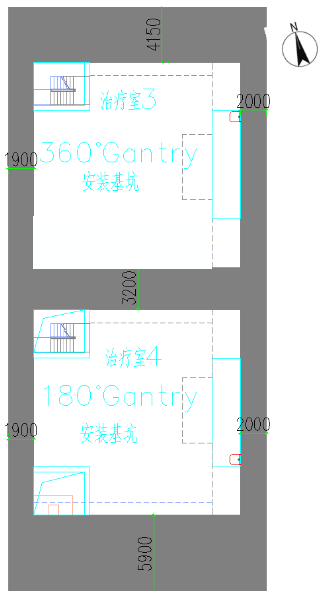
图 4.1.1-5 质子重离子机房辐射屏蔽设计（负一层）
