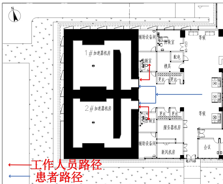
图 3.2.2-6 电子直线加速器人员路径图
