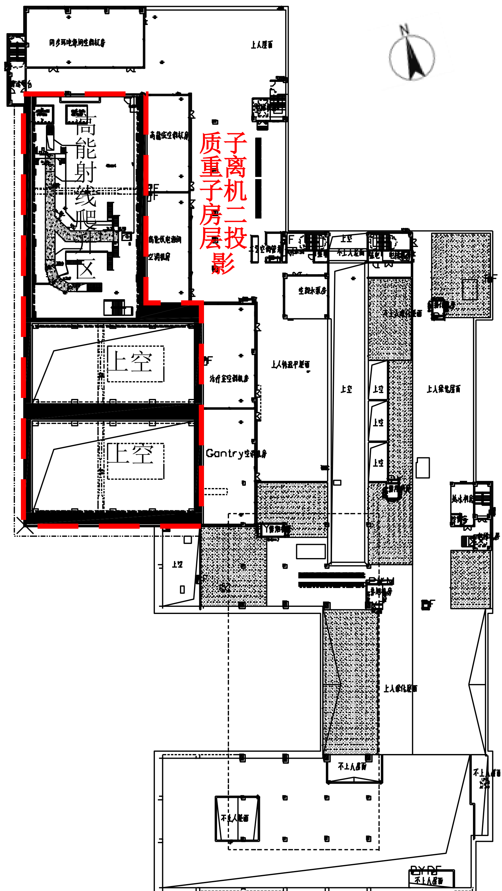
图 1.2.5-8 重离子质子中心三层平面布置图
