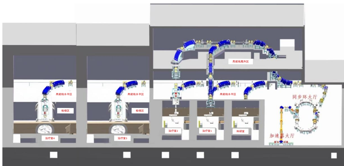
图 3.2.1-2 质子重离子一体化治疗系统总体布局示意图
