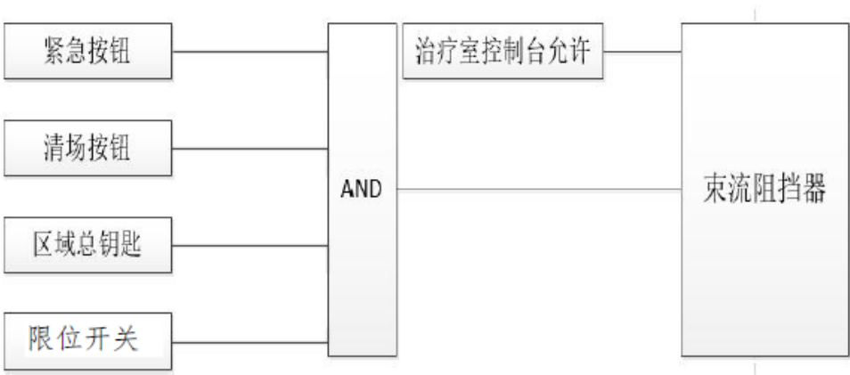
图 4.1.2-16 治疗室出束联锁逻辑图
