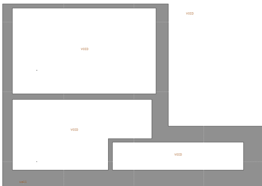
图 5.2.2-2 FLUKA 计算模型（科研室、治疗室 1-2 剖面图）
