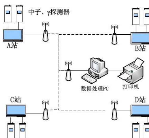
图 4.1.2-11 环境辐射监测系统组成
