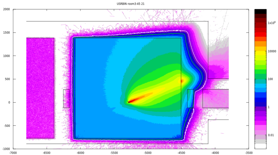
图 5.2.2-11 45° 照射时，质子重离子机房剂量率分布图， \mu\text{Sv/h}
