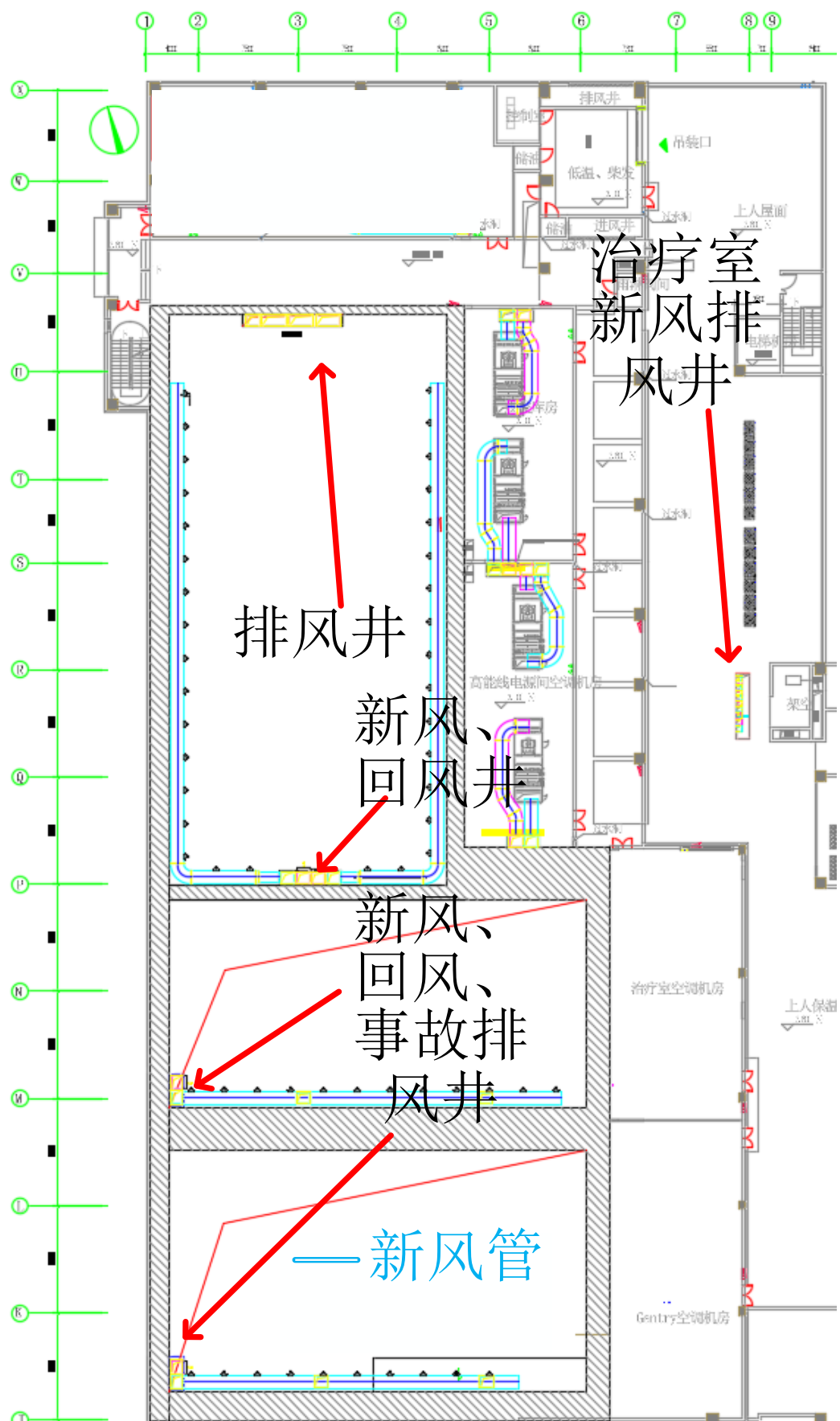
图 4.1.2-19 质子重离子机房通排风管道示意图（三层）
