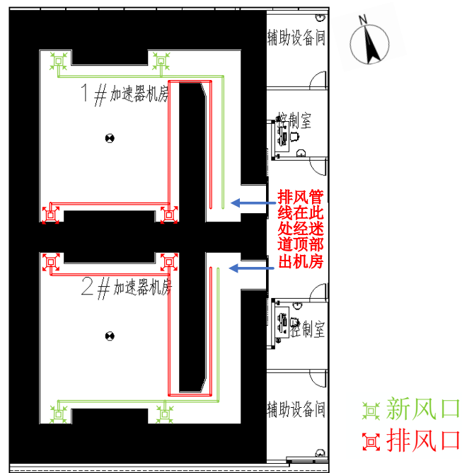
图 4.2.3-2 加速器机房通排风示意图
