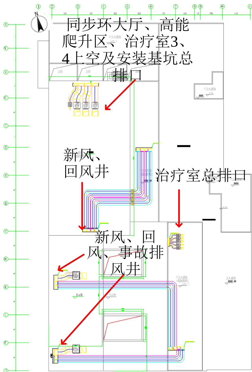
图 4.1.2-20 质子重离子机房总排气口位置示意图（屋顶层）
