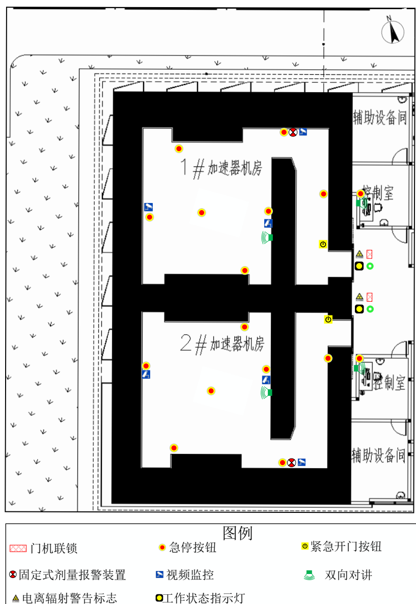
图 4.2.2-1 加速器机房急停按钮、监视系统等安全设施分布示意图
