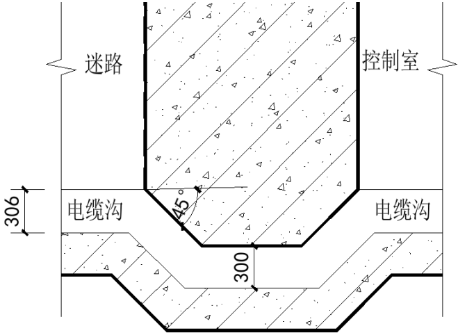
图 4.2.3-3 加速器机房电缆穿墙示意图
