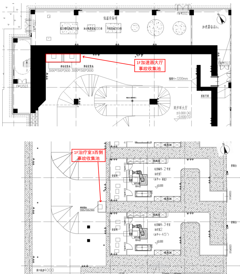
图 4.1.3-1 事故收集池和放射性废物间位置示意图
