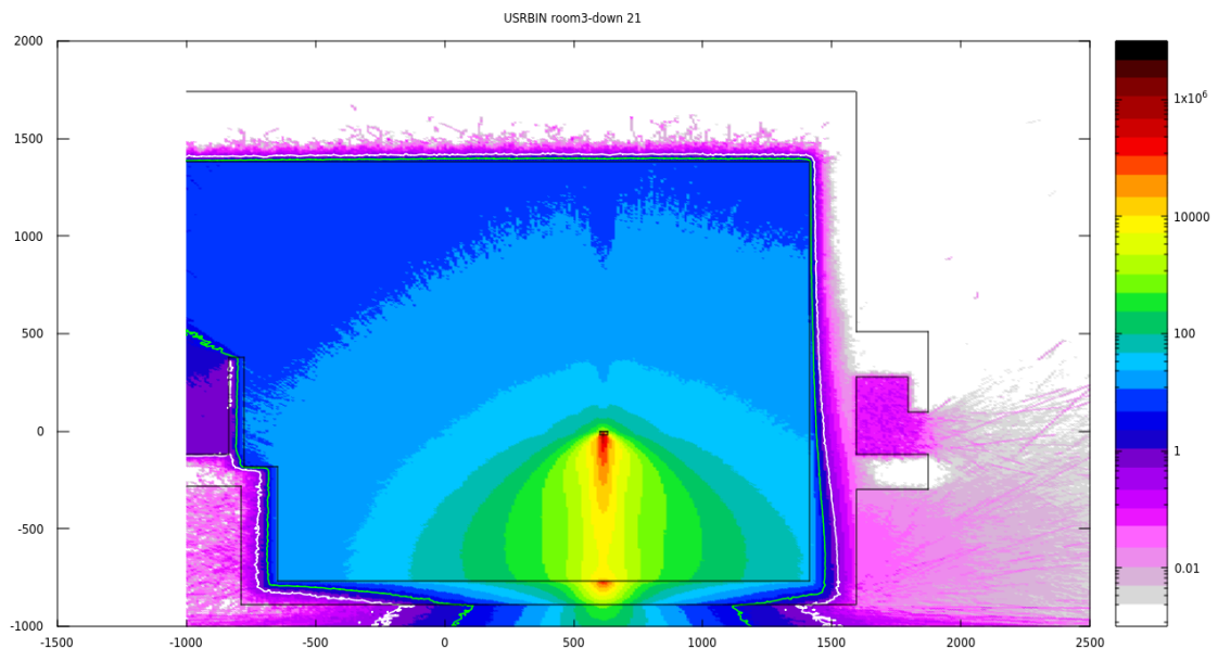
图 5.2.2-12 朝地面照射时，质子重离子机房剂量率分布图， \mu\text{Sv/h}
