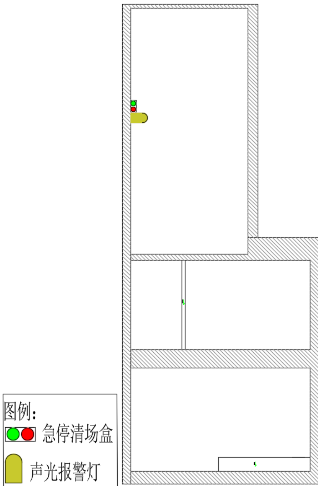
图 4.1.2-13 质子重离子机房内安全联锁设施安装点位（二层）
