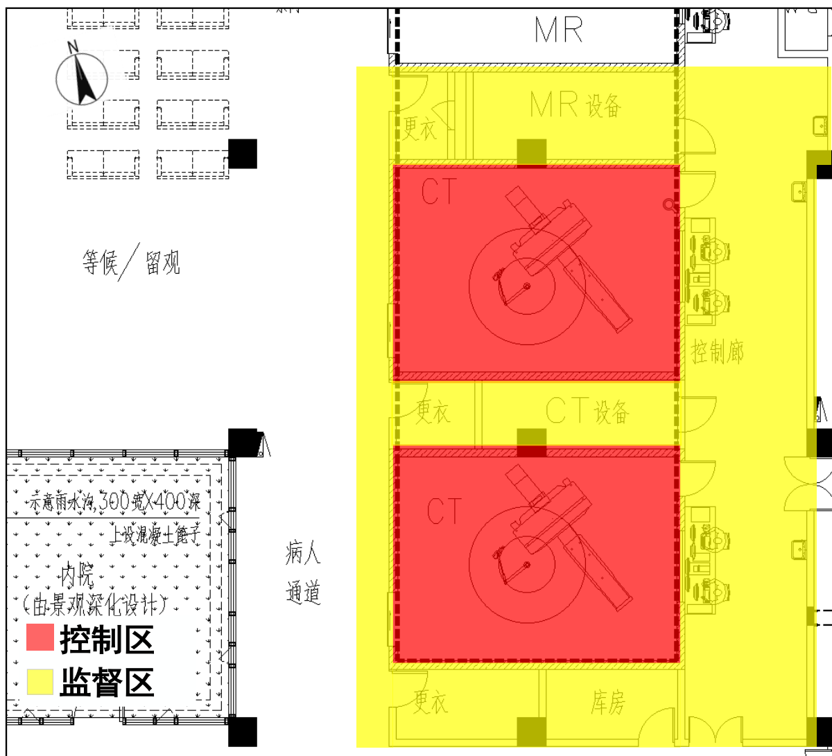
图 4.3.1-1 模拟定位 CT 辐射工作场所分区图
